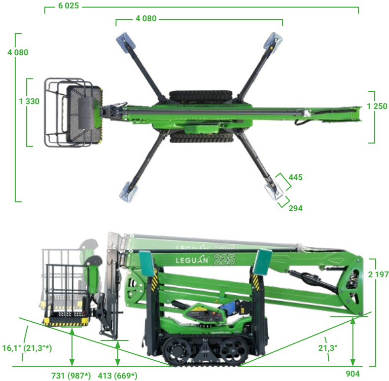
Matuojama milimetrais. *Pakeltos vairavimo padėties (EDP) maksimalūs rodikliai.
