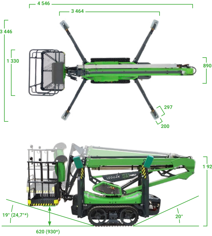
Matuojama milimetrais. *Pakeltos vairavimo padėties (EDP) maksimalūs rodikliai.
